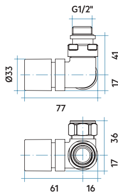
Válvula
